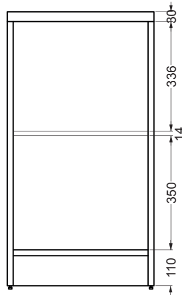
VISTA FRONTALE SENZA ANTA
