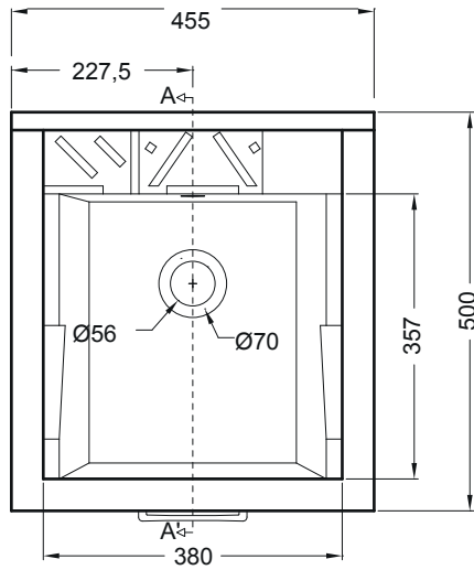
PIANTA
