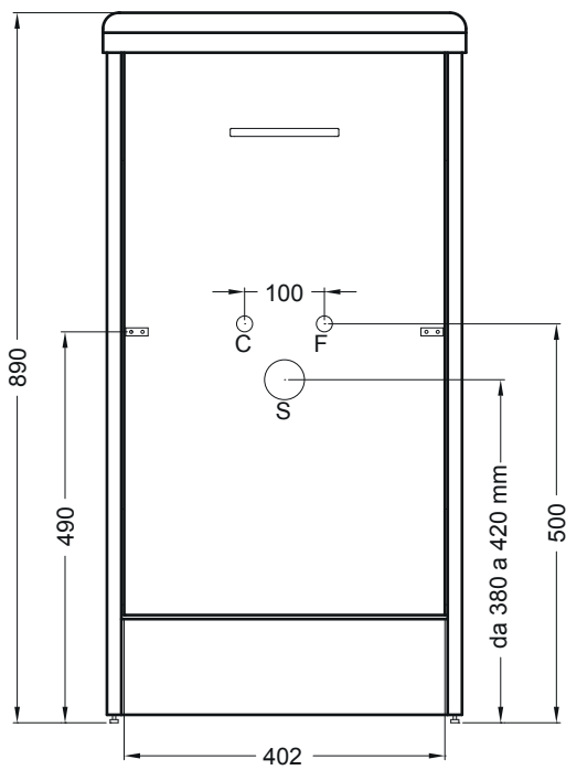
VISTA FRONTALE
