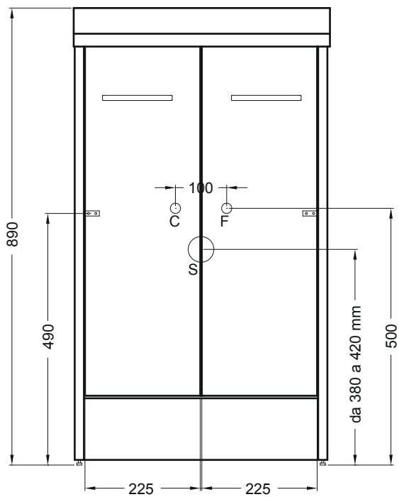
VISTA FRONTALE
