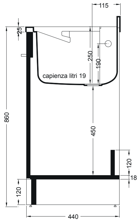
SEZIONE A-A
